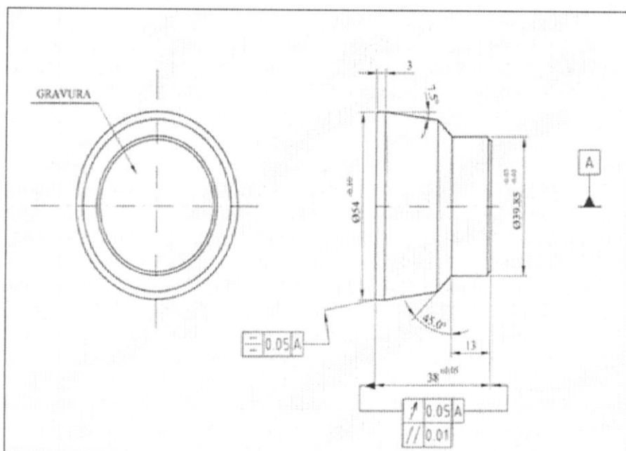
Слика 12 : Технички цртеж ковачког алата за медаље
