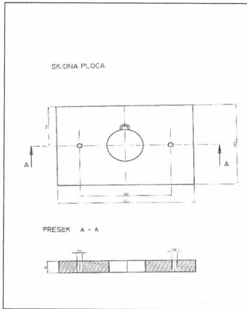
Слика 24: Технички цртеж скидне плоче
