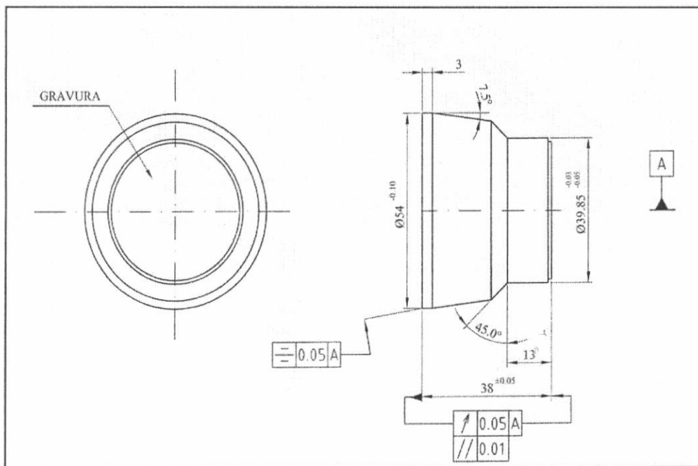
Слика 2: Технички цртеж ковачког алата за медаље
