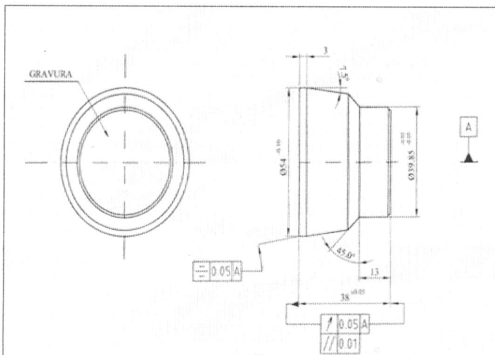
Слика 16: Технички цртеж ковачког алата за медаље
