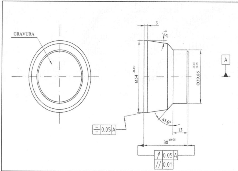
Слика 8: Технички цртеж ковачког алата за медаље
