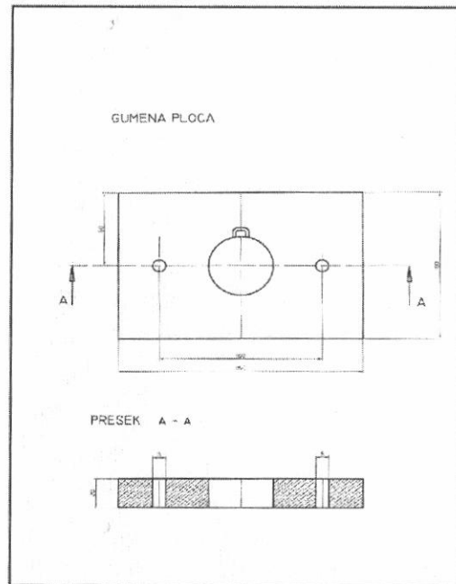
Слика 25: Технички цртеж гумене плоче
