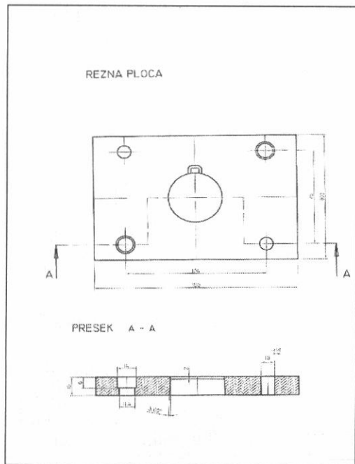
Слика 17: Технички цртеж резне плоче
