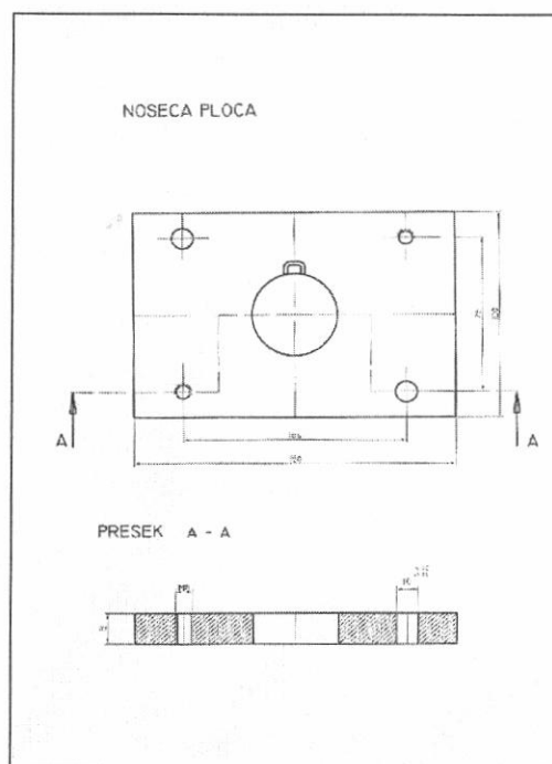
Слика 23: Технички цртеж носеће плоче
