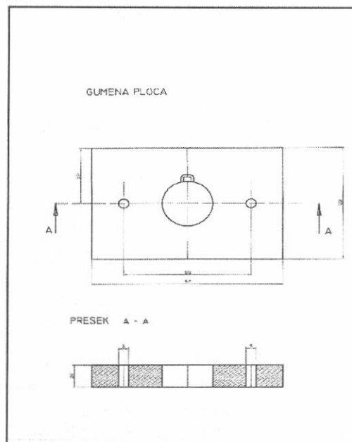
Слика 20: Технички цртеж гумене плоче
