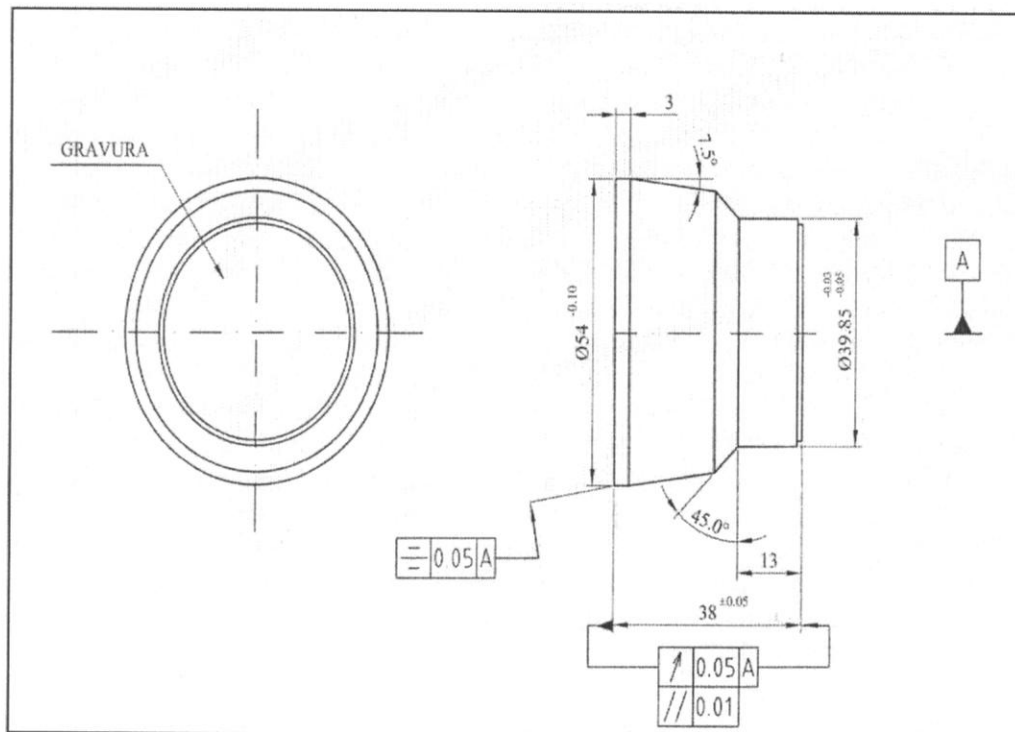
Слика 6: Технички цртеж ковачког алата за медаље
