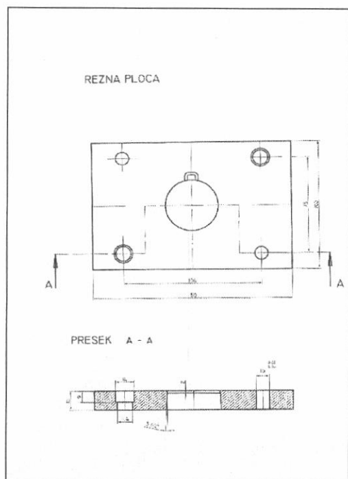
Слика 22 Технички цртеж резне плоче
