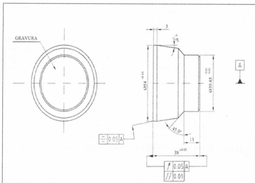
Слика 10 : Технички цртеж ковачког алата за медаље
