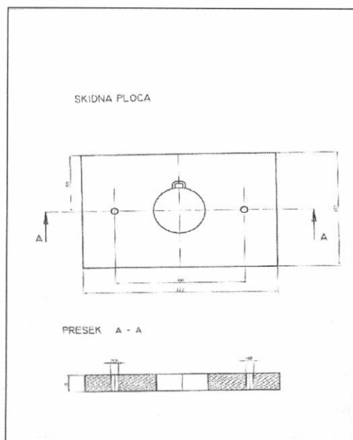
Слика 19: Технички цртеж скидне плоче
